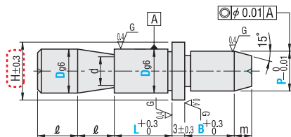
全周溝形状
